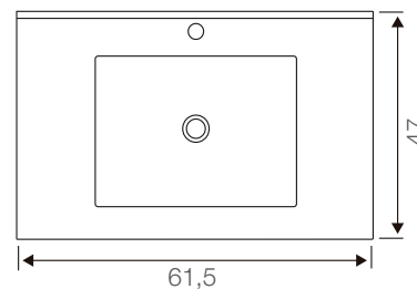
Dimensiones Cubierta
